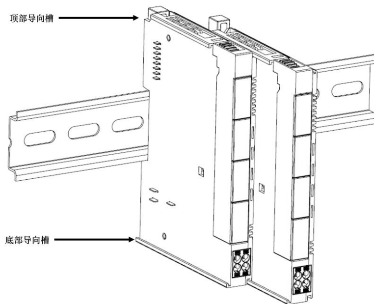
图 6 模块导向槽示意图
