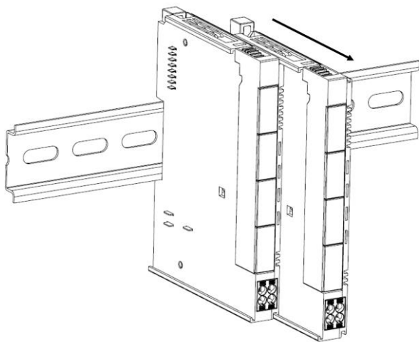
图 10 拉出模块示意图
