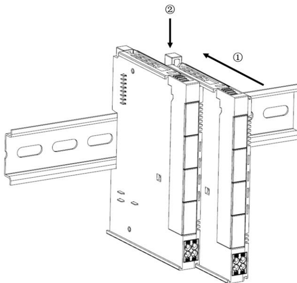
图 7 模块安装示意图
