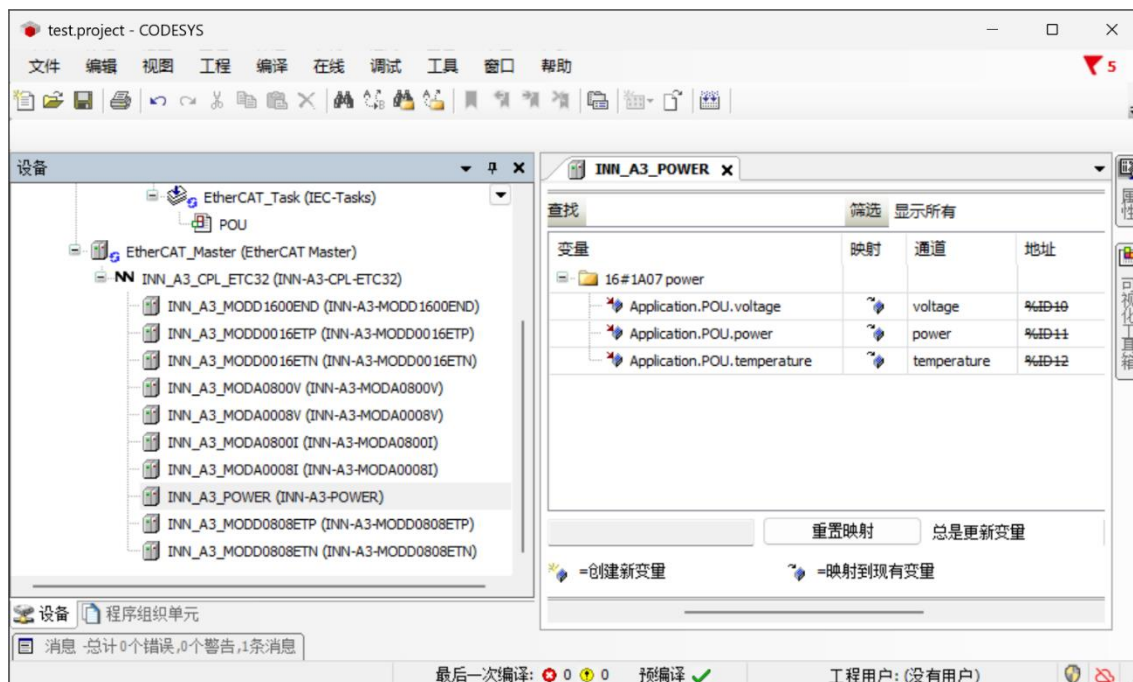
图 17 设置映射
