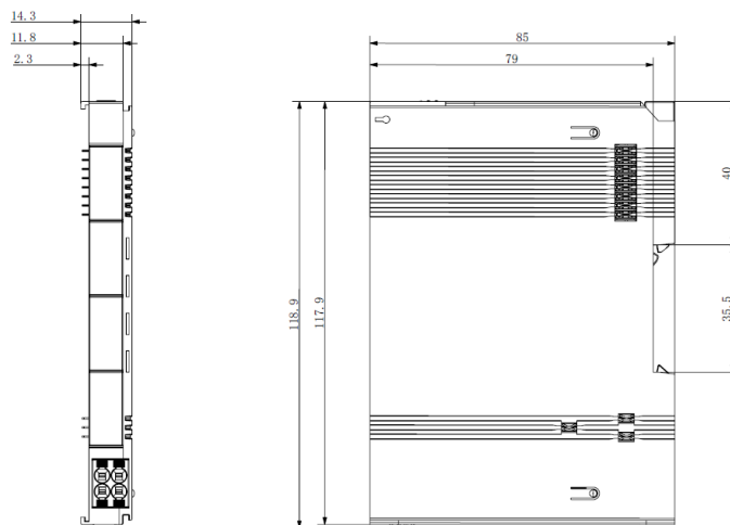
图 4 模块尺寸图
