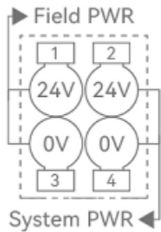
图 3 端子接线图
