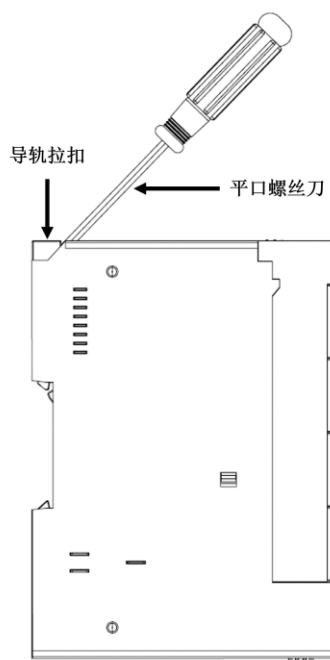
图 9 撬动导轨锁扣示意图
