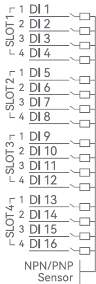
图 3 端子接线图
