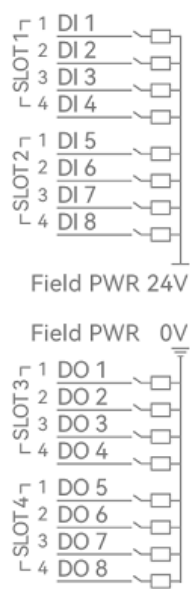
图 3 端子接线图
