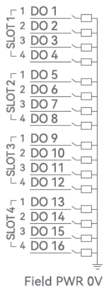
图 3 端子接线图
