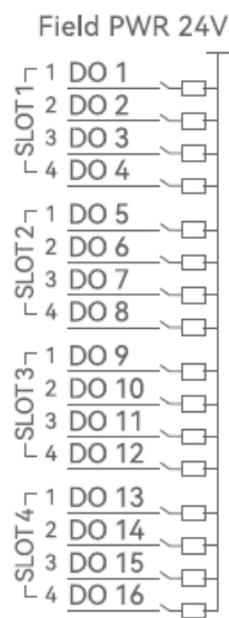
图 3 端子接线图
