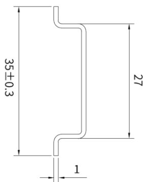
图 5 DIN 导轨图
