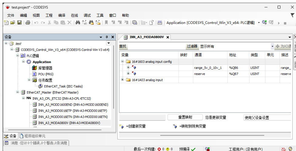
图 18 设置量程
