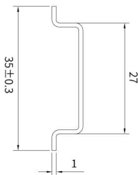
图 5 DIN 导轨图
