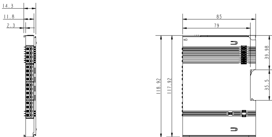
图 4 模块尺寸图
