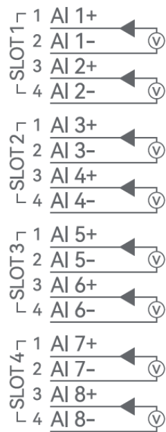
图 3 端子接线图
