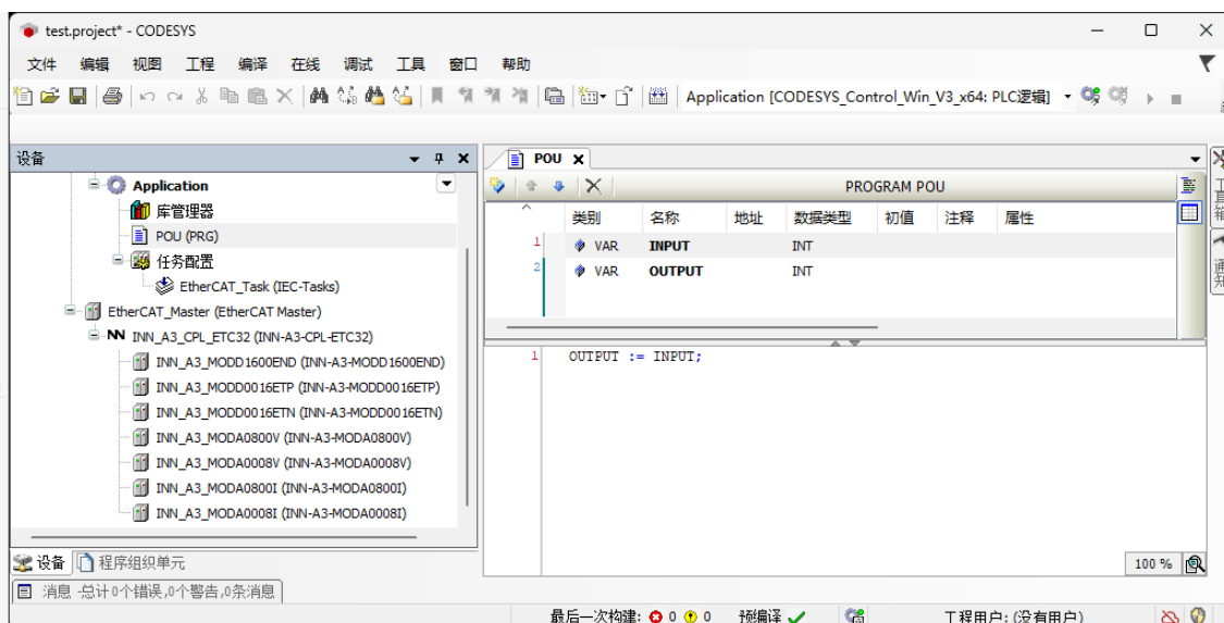
图 16 代码窗口
