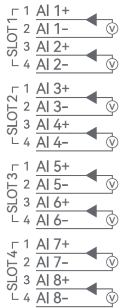
图 3 端子接线图
