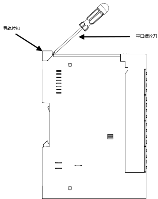
图 9 撬动导轨锁扣示意图
