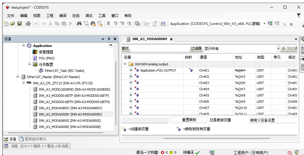
图 17 设置映射
