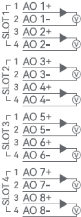
图 3 端子接线图
