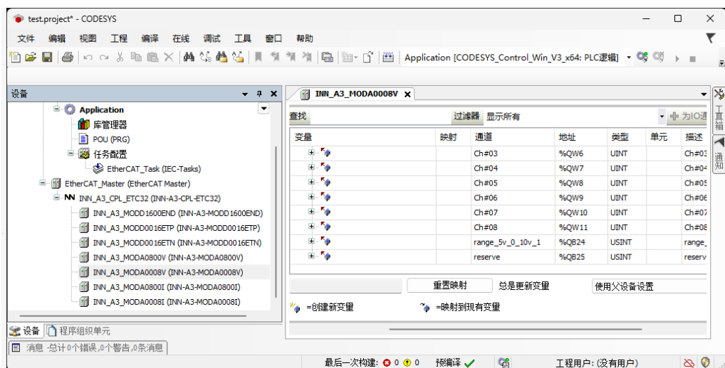
图 18 设置量程
