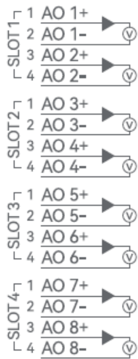
图 3 端子接线图
